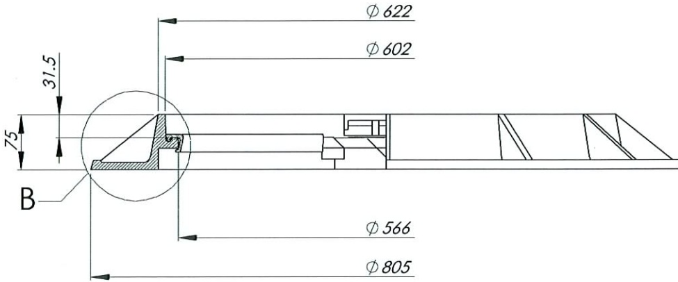
Secção: A-A
