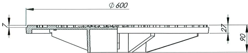
Secção: A-A
