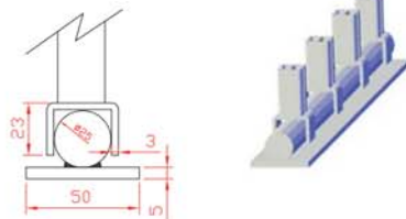
Guia inferior especial Vergalhão aparafusado
