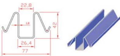
Guia inferior especial Vergalhão aparafusado
