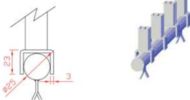
Guia inferior especial Vergalhão chumbado
