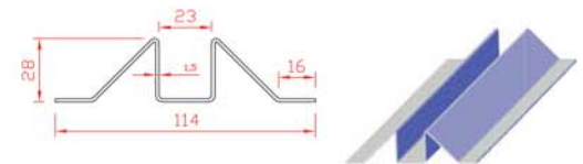
Guia inferior especial aparafusada
