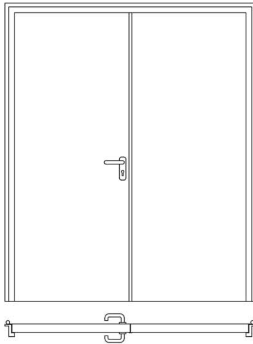
Duas folhas
