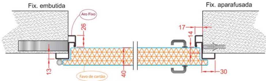
Fixação
