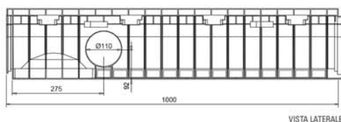
VISTA LATERALE
