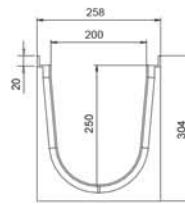
SEZIONE
