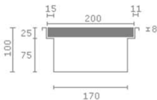
Perfil Canal modular p/grelha L200 (exemplo dadas as variações possíveis)
